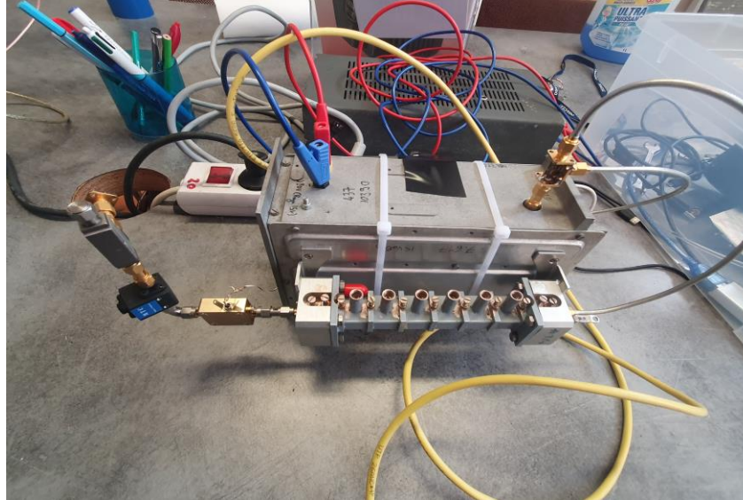
L'émetteur 10 GHz(Pluto+ Ol + Filtre)
